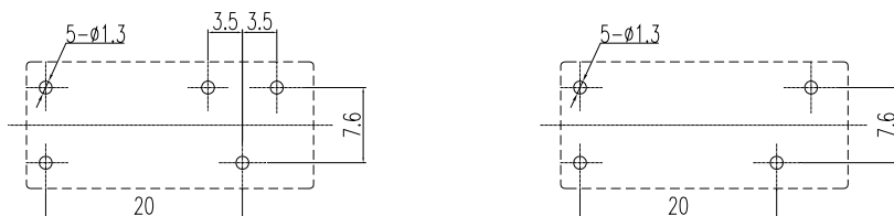
安装孔位图 (底视图)
